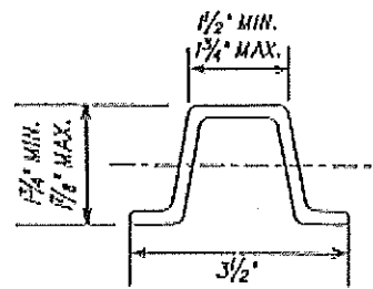
A-A SECTION
